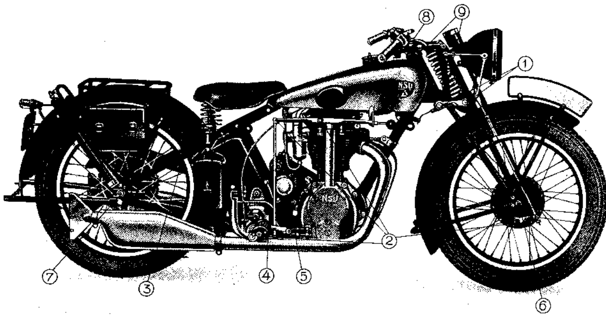
Abb. 14 — Schmierplan
