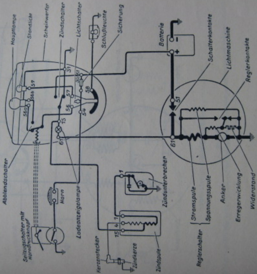
Bild 67 Kraftanlage mit Gleichstrom-Lichtmaschine, Batterie und Scheinwerfer (E/MTA 160)
