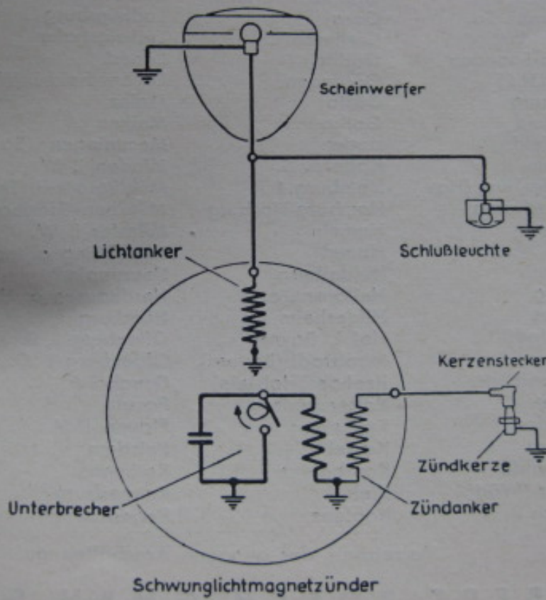
Bild 10 Schaltbild einer Kraft- anlage mit Schwunglichtmagnet- zünder LM/UT 1/142/30
